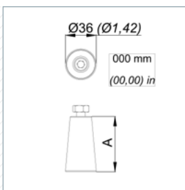
SUA001/ SUA901 (FINGER FOR BJH OR SUA002)
