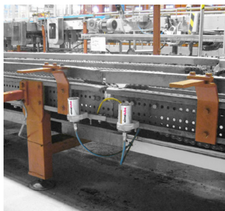
Dve maznice simalube s predlžovacími hadicami premazávajú prenosovú reťaz v pivovare.
